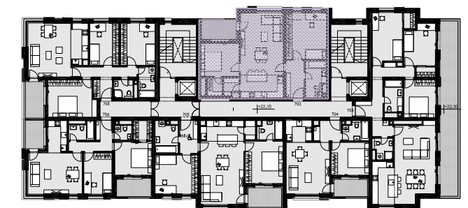
ETAŽA +7
